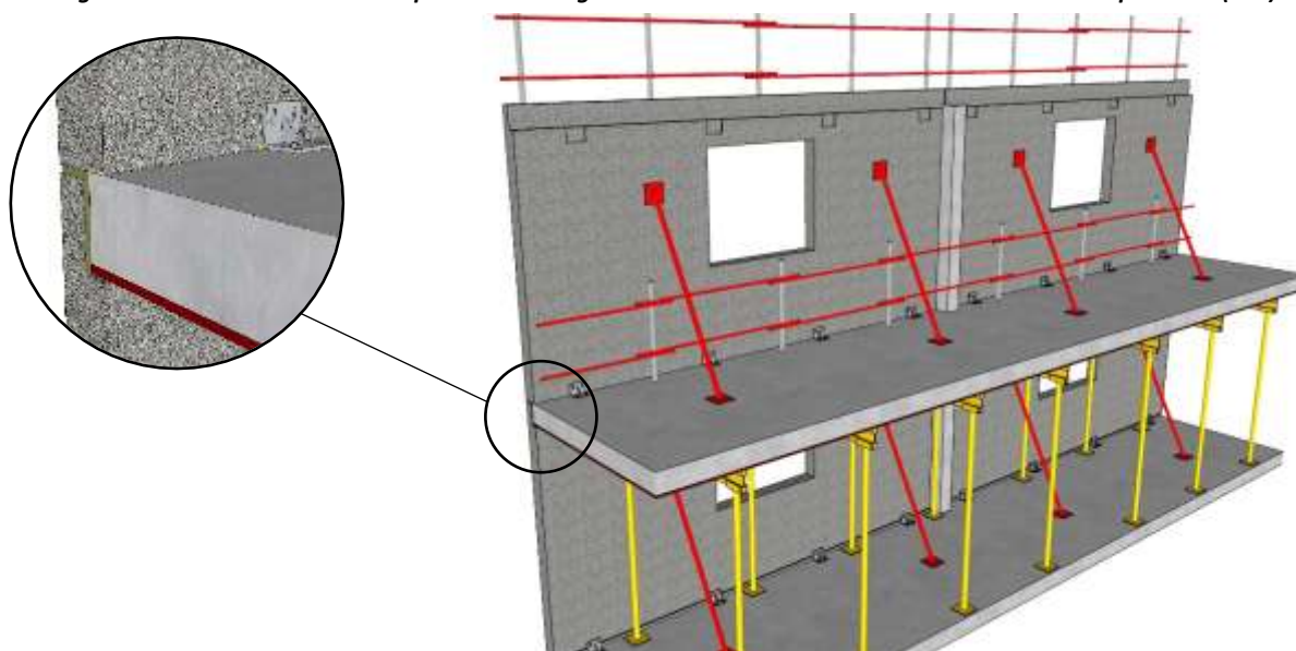
Figure 21 – Pose des panneaux des étages suivants (FP3)
