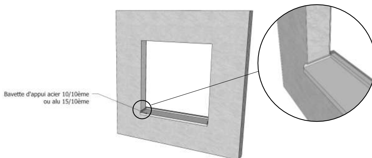
Figure 32 – Mise en œuvre de la bavette d'appui
