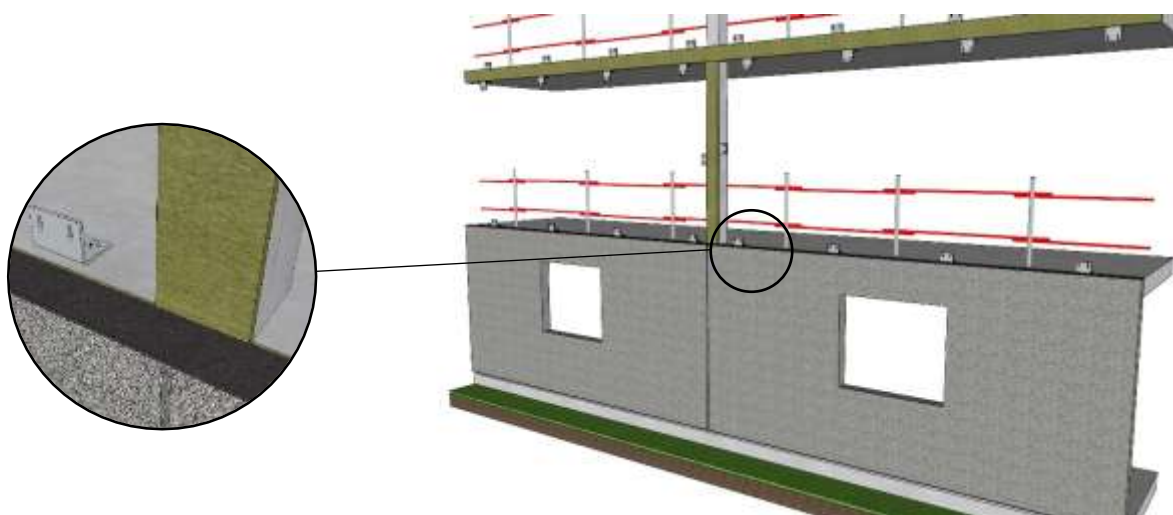
Figure 10 – Mise en œuvre du mortier sur le chant supérieur des panneaux (FP2)
