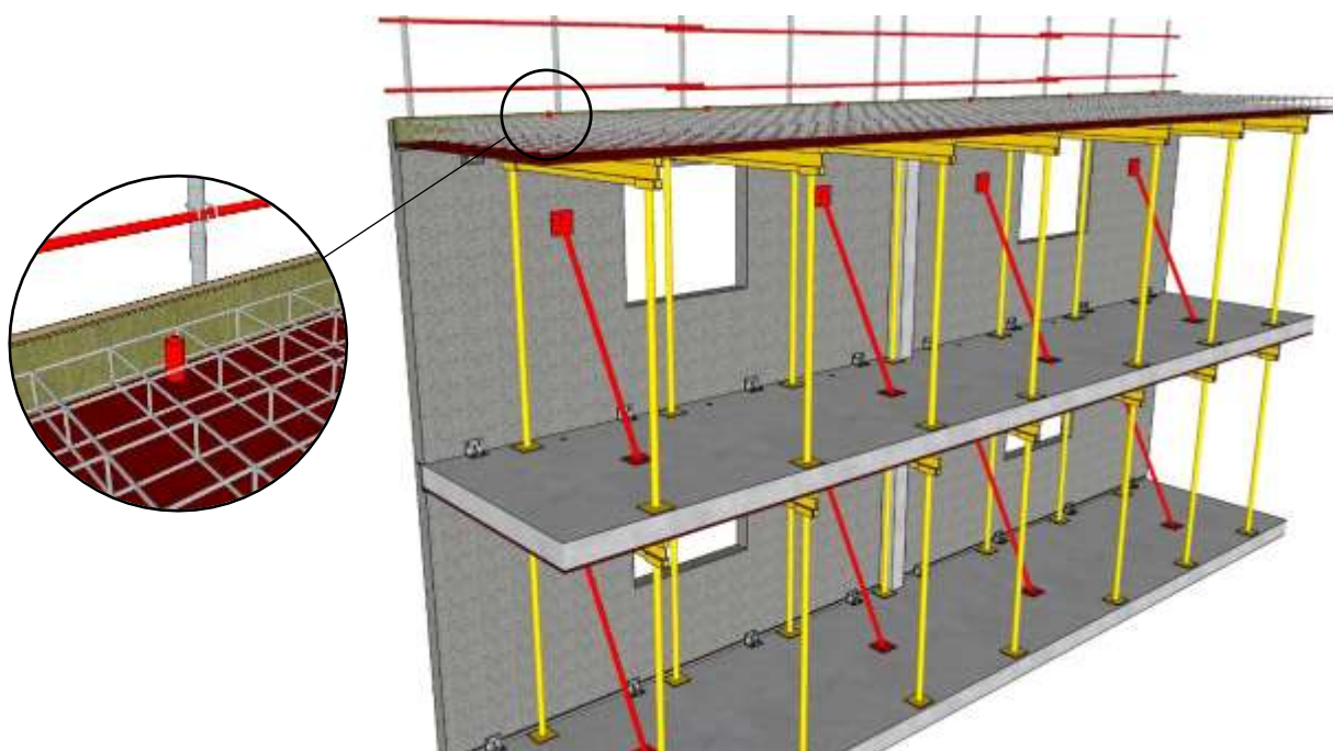
Figure 23 – Pose des armatures métalliques et ligature avec les fers à béton pliés des équerres d'ancrage. Intégration des douilles pour pieds de garde-corps en bord de dalle (FP3)
