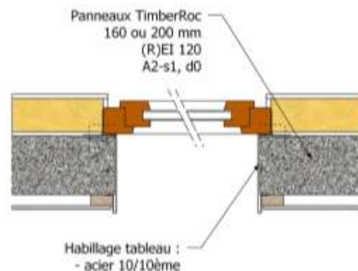
Coupe horizontale
