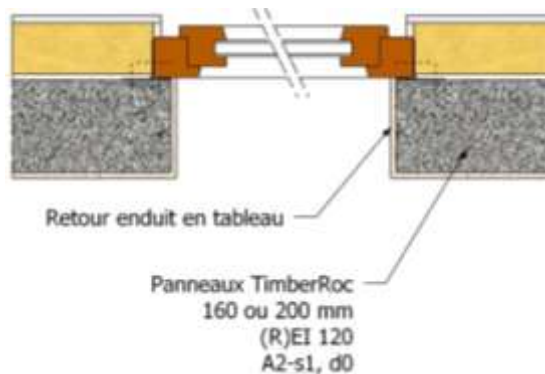
Coupe horizontale
