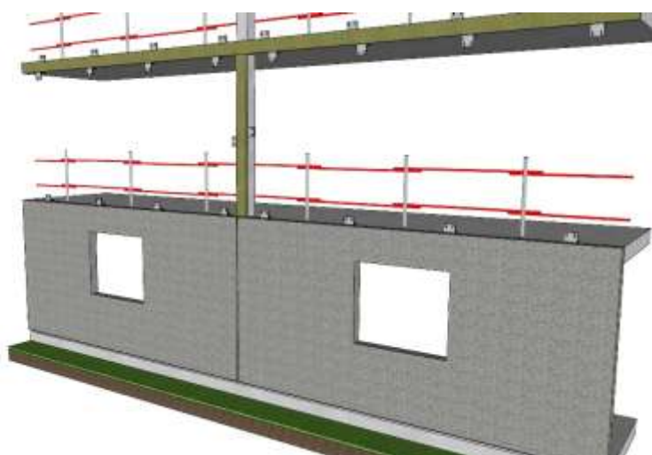
Figure 8 – Mise en place des panneaux suivants (FP2)
