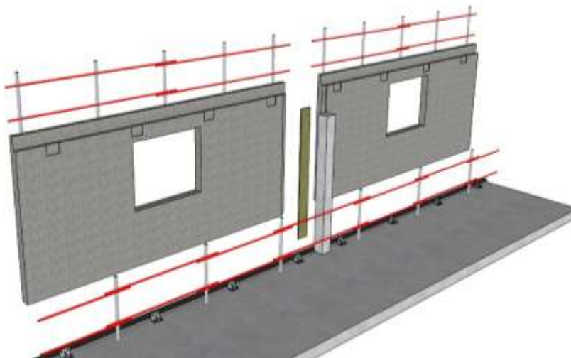
Figure 15 – Vue des panneaux de façade en approche (FP3)
