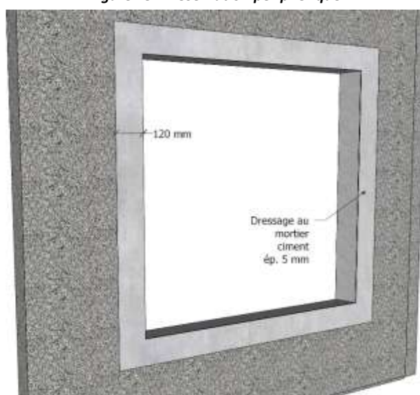
Figure 26 – Dressage au mortier ciment
