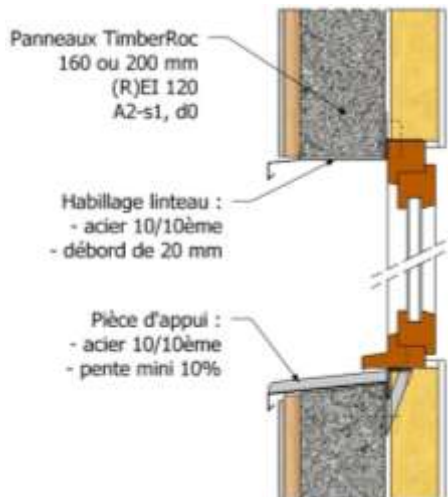
Coupe verticale
