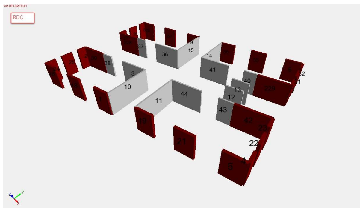
Fig. 15 – Modèle mixte (béton en gris et CS2 en rouge) – Vue RDC avec nomenclature
