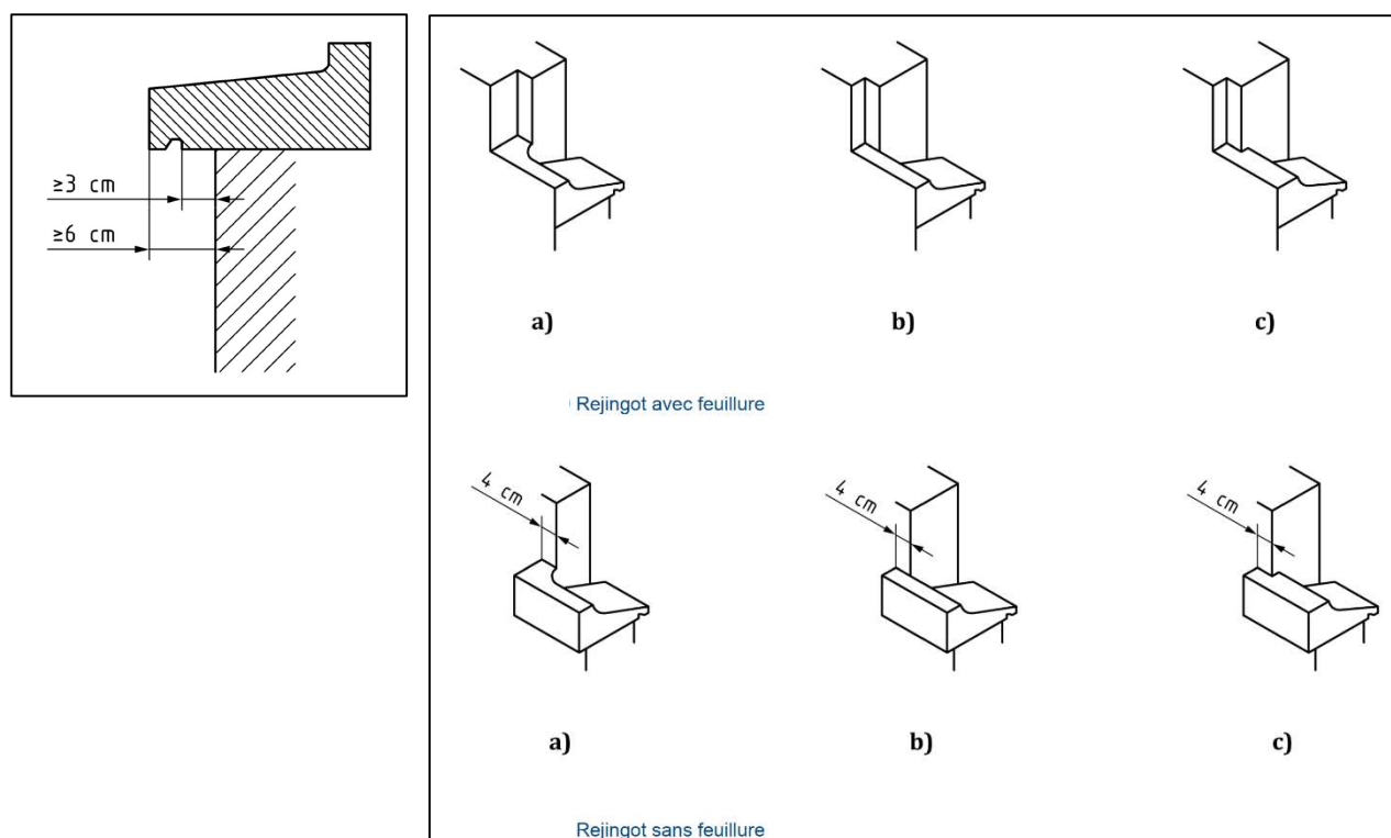
Figure A33 : Appuis de baies en béton
