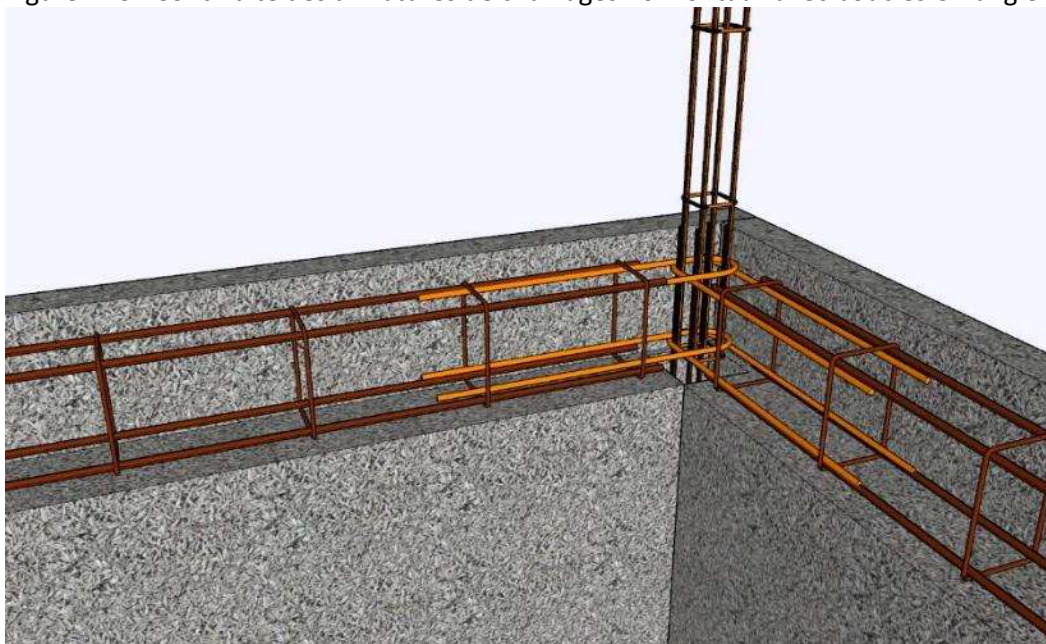
Figure A13 : Continuité des armatures de chaînages horizontaux avec boucles U - angle
