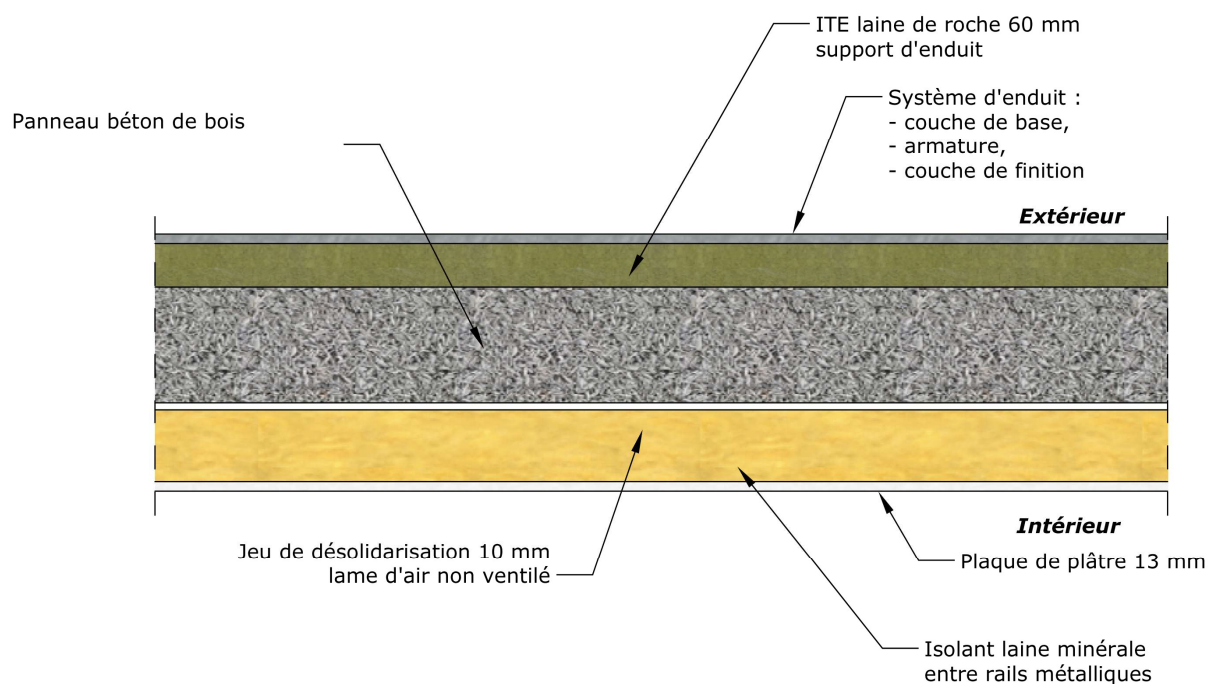
Figures A41 : Exemple partie courante Panneau avec ETICS
