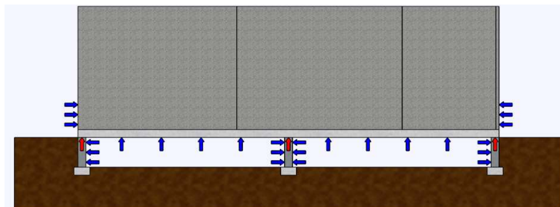
Figure A05 : Protection contre les termites – schéma de principe avec parois contrôlables
