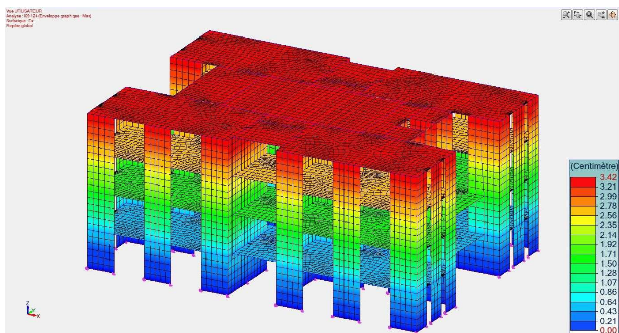
Fig. 11 – Modèle béton de bois CS2 – Déformée Dx selon direction X
