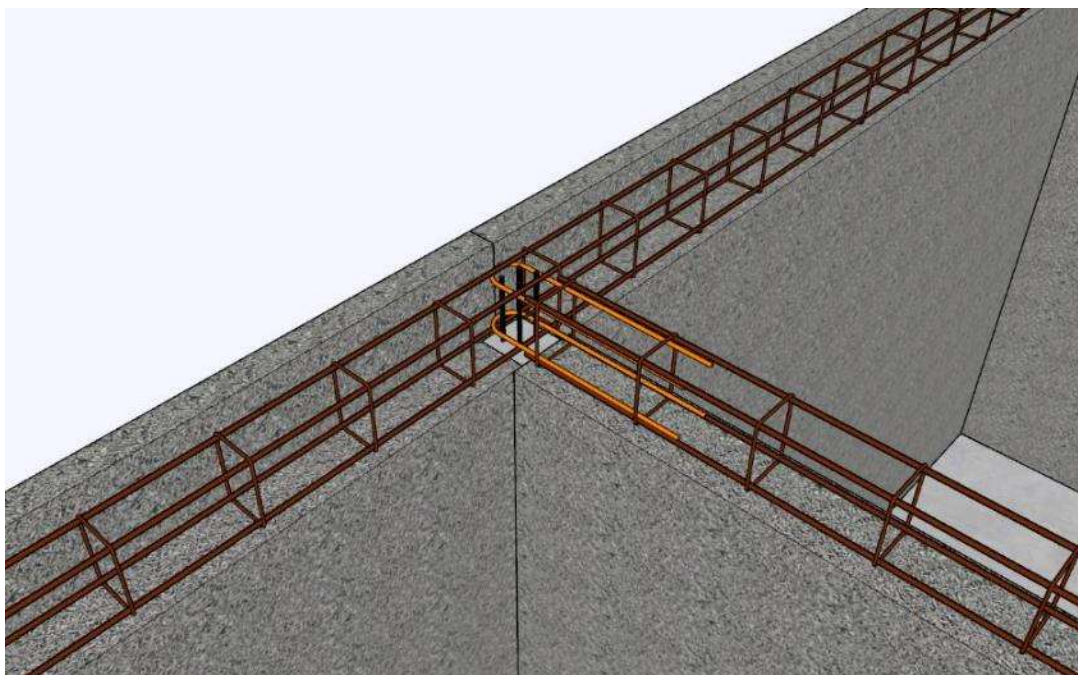
Figure A15 : Continuité des armatures de chaînages horizontaux avec boucles U – Liaison refend / vue perspective
