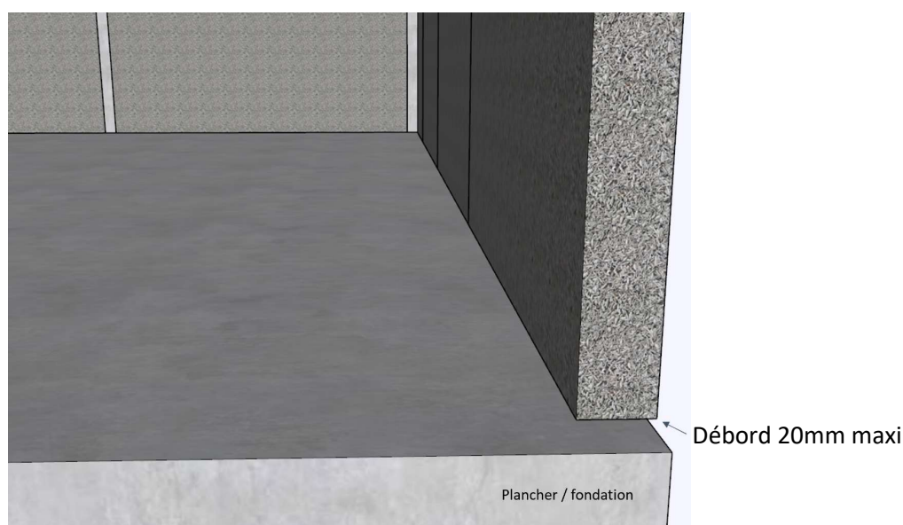
Figure A01 – Débord assise des murs TimberRoc
