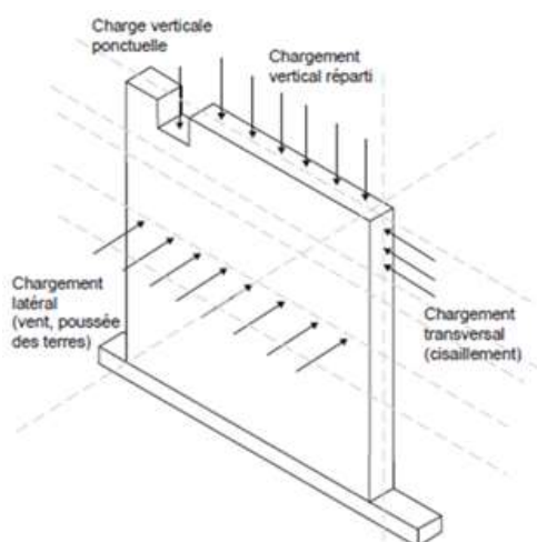
Figure A07-1 : Types de chargement appliqués sur les murs en panneaux TimberRoc
