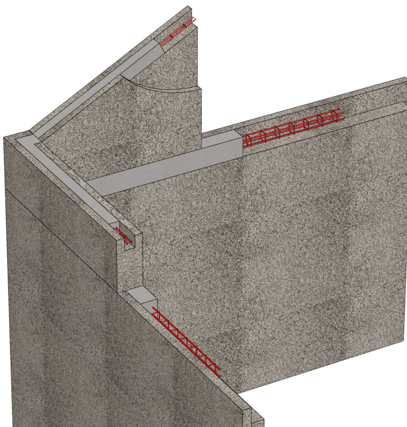
Figure A21 : Visuel principe chaînage rampant
