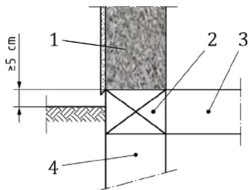
Figure A04 : Disposition anti-capillarité – solution 2 avec soubassement en béton armé
