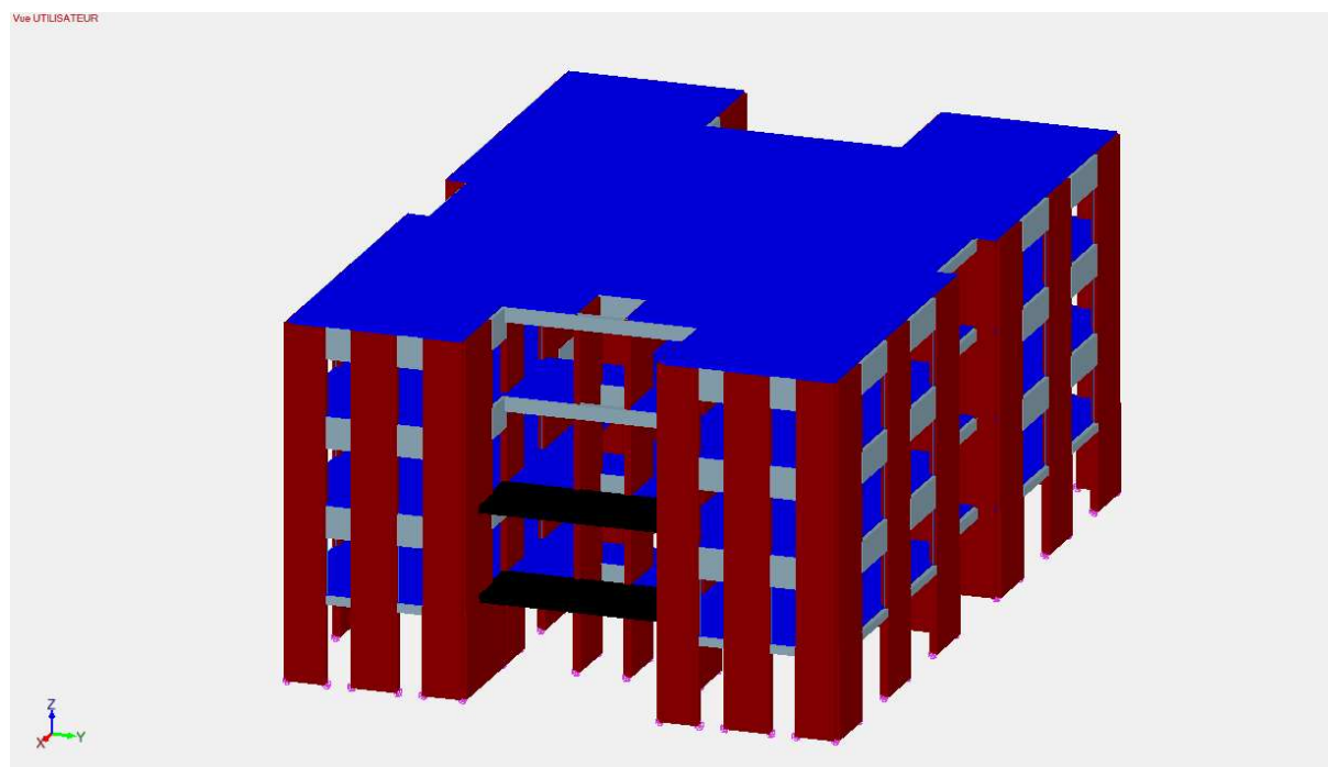
Fig. 7 – Modèle béton de bois CS2 - Axonomie 3
