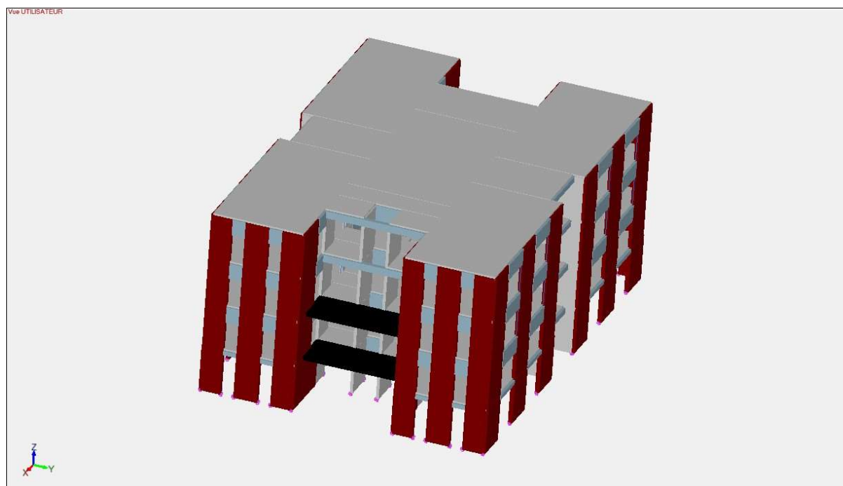
Fig. 14 – Modèle mixte (béton en gris et CS2 en rouge) - Axonométrie 3
