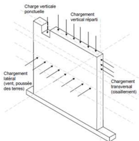
Figure A07-1 : Types de chargements appliqués sur les murs
