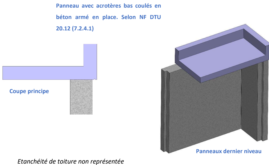
Figure A24-B : Acrotère bas intégré au panneau CS2
