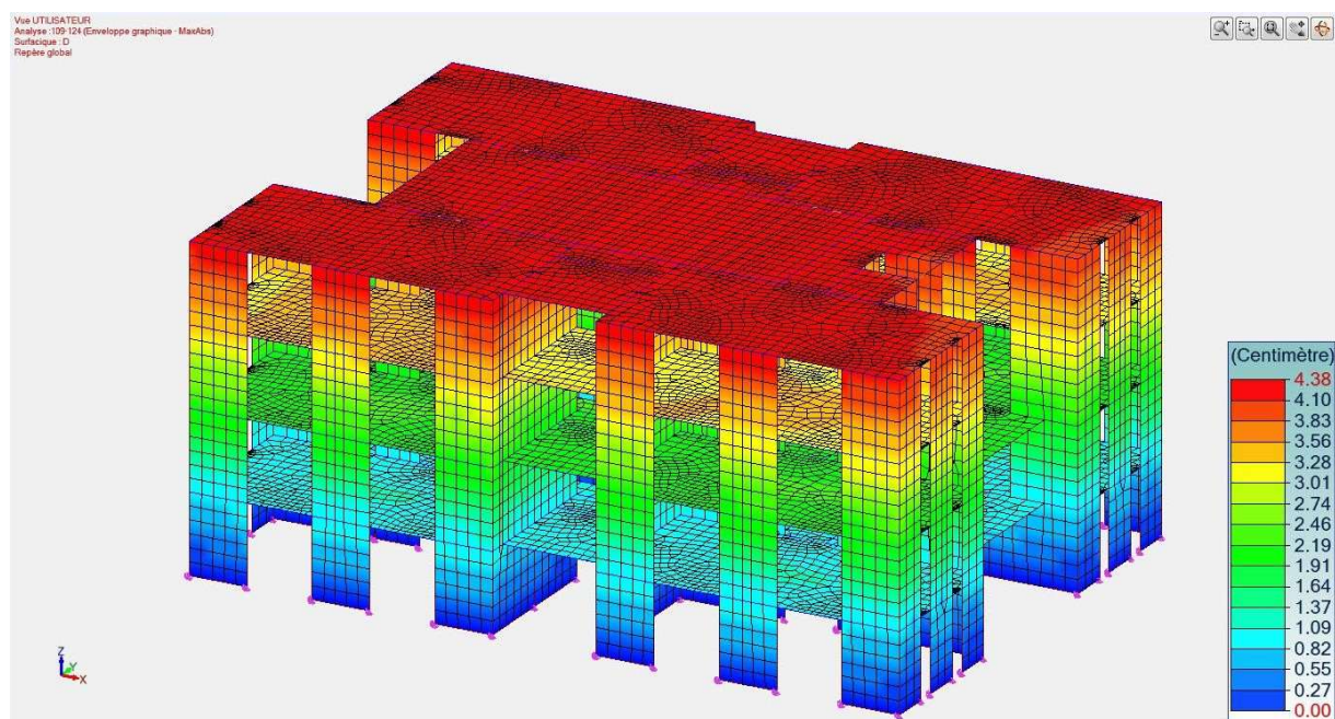
Fig. 10 – Modèle béton de bois CS2 – Déformée globale D
