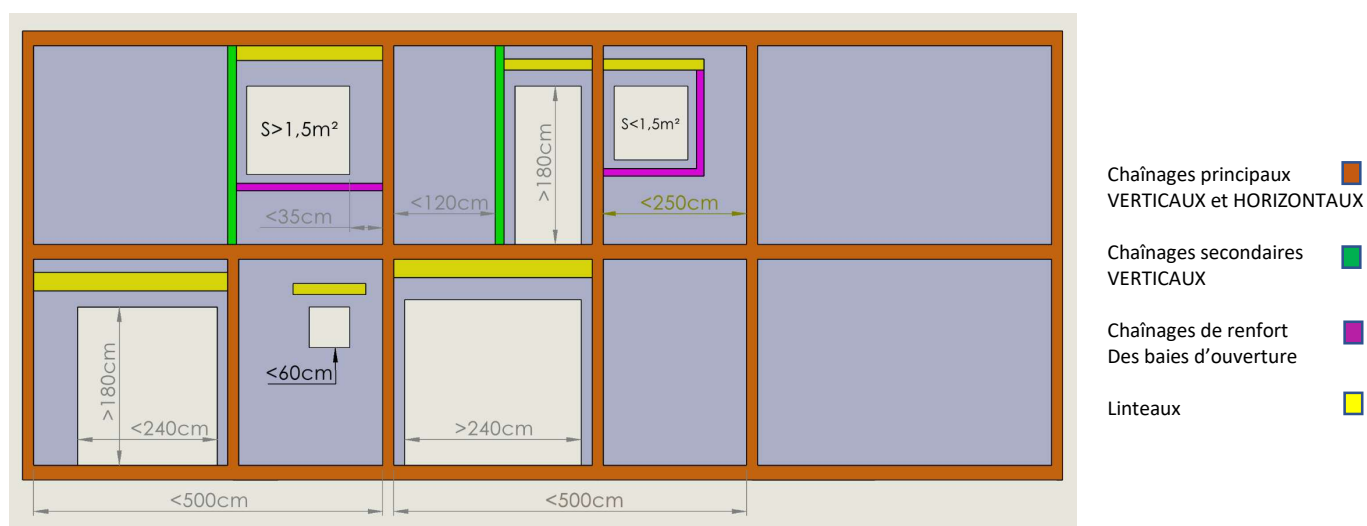
Figure A28 : Dispositions de principe des chaînages pour les configurations B et C, zones sismiques 3 et 4 – hors analyse de structure :
