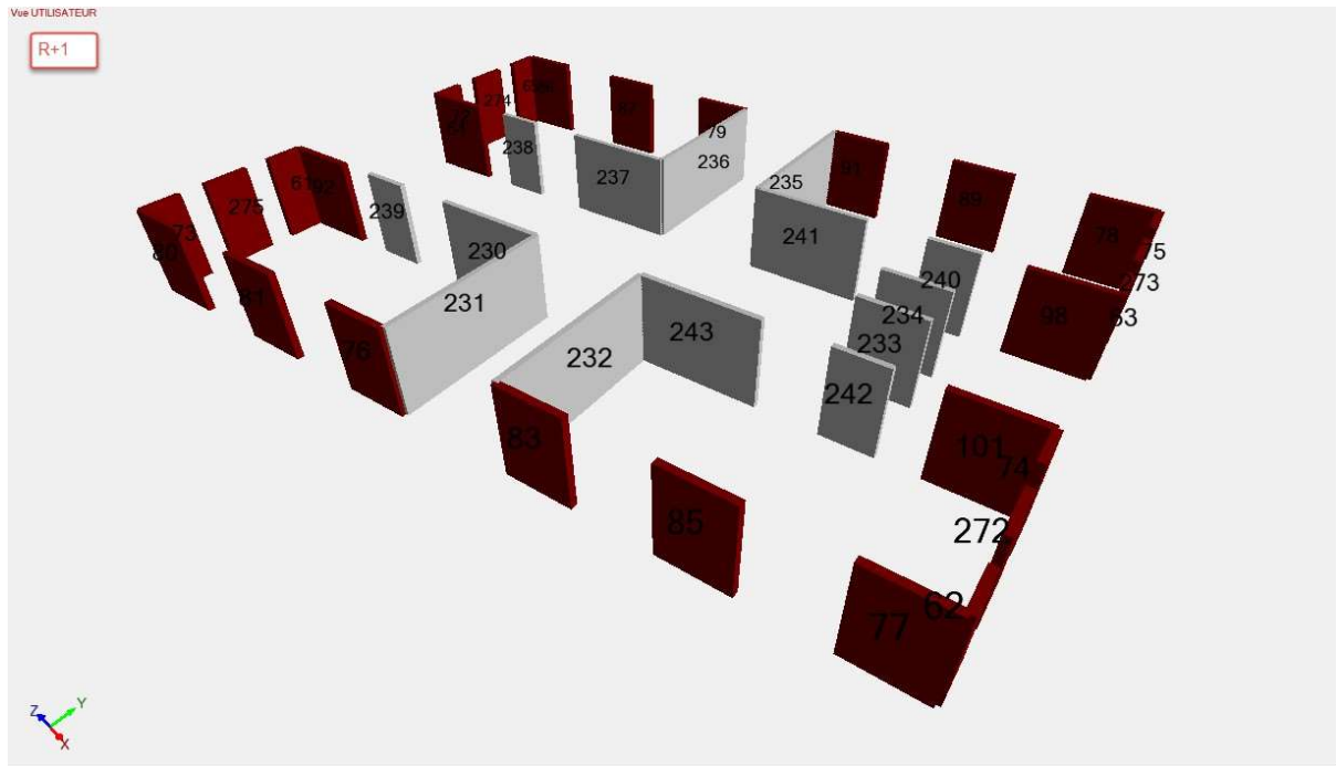
Fig. 16 – Modèle mixte (béton en gris et CS2 en rouge) – Vue R+1 avec nomenclature
