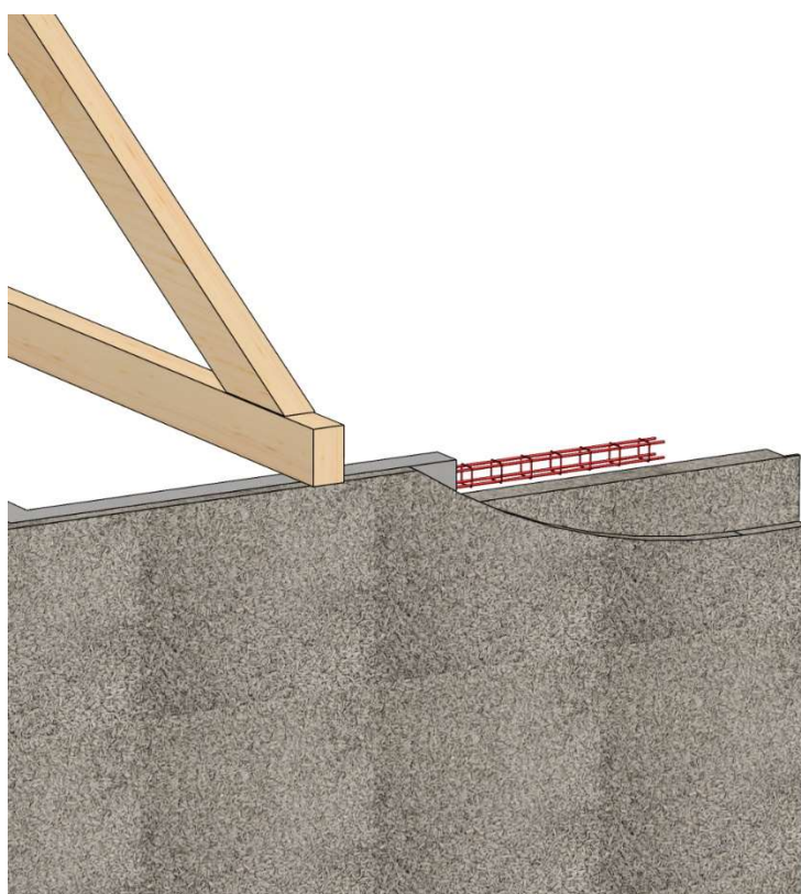
Figure A23 : Appui d'une ferme de charpente sur une semelle de répartition (chaînage)
