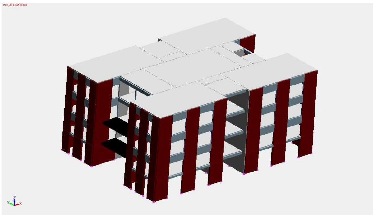
Fig. 12 – Modèle mixte (béton en gris et CS2 en rouge) - Axonométrie 1
