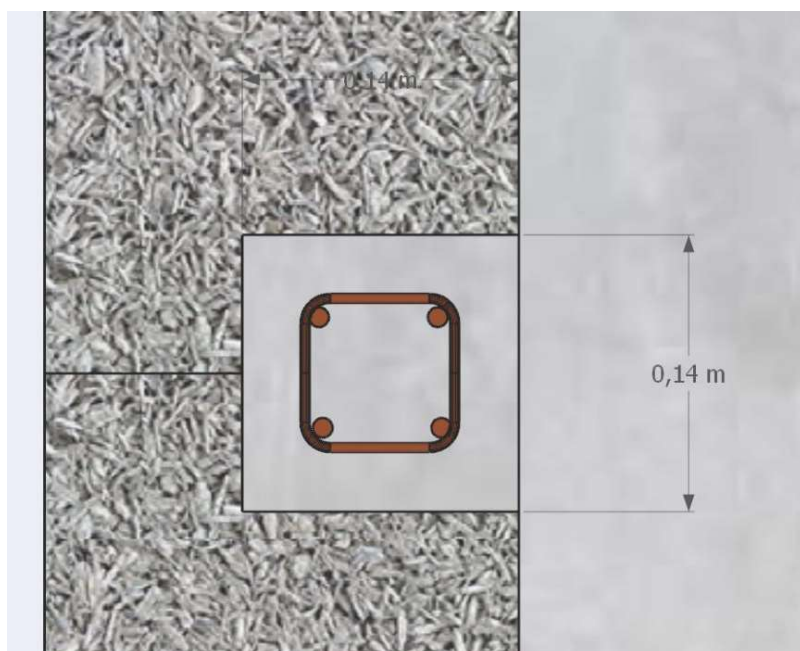
Figure A09 : Vue de principe en coupe d'un chaînage vertical Principal
