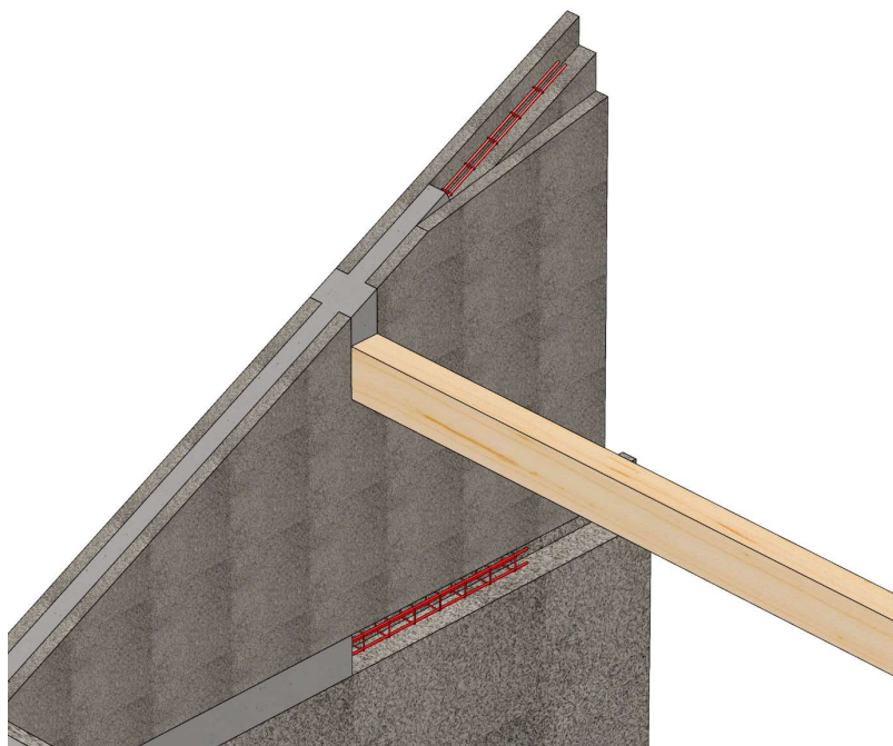
Figure A23 : Appui d'une ferme de charpente sur une semelle de répartition (chaînage)
