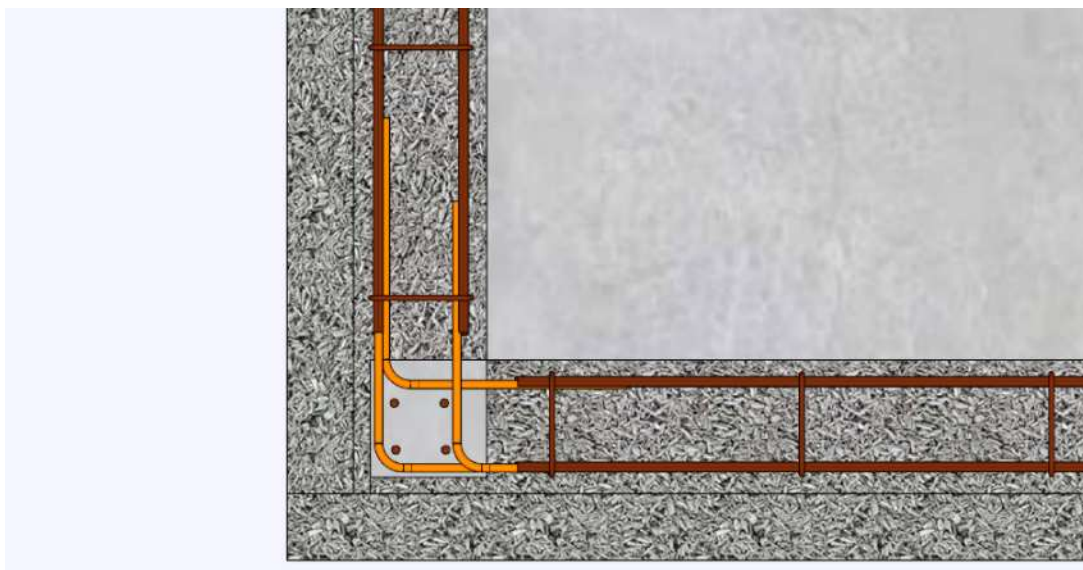
Figure A16 : Continuité des armatures de chaînages horizontaux avec équerres- angle
