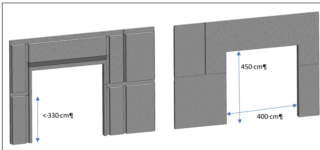
Figure A35 : Exemple de réalisation d'une porte sectionnelle de grandes dimensions
