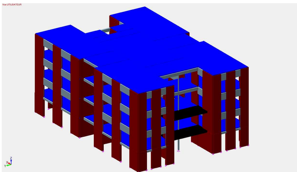
Fig. 6 – Modèle béton de bois CS2 - Axonométrie 2
