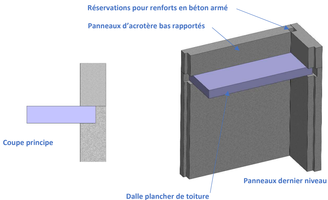
Figure A24-D : Acrotère bas rapporté sur dalle toiture
