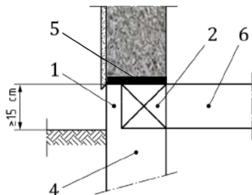
Figure A03 : Disposition anti-capillarité – solution 2 avec chappe de mortier hydrofuge si soubassement en maçonnerie
