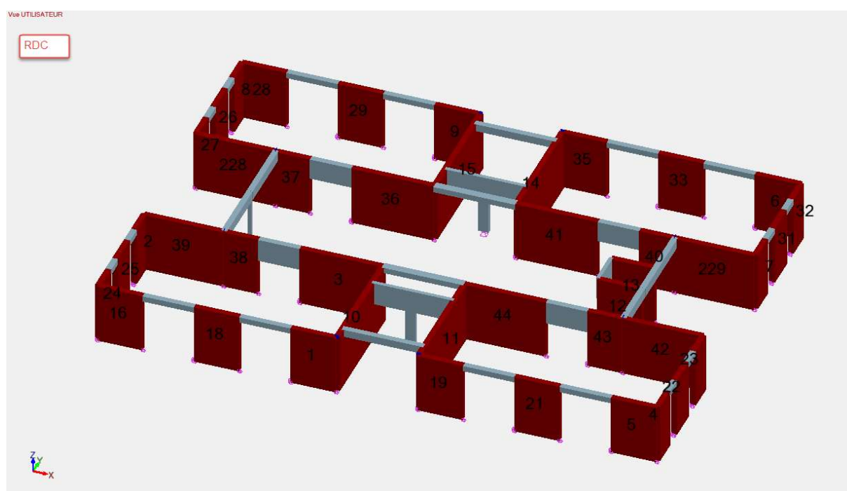
Fig. 8 – Modèle béton de bois CS2 – Vue RDC avec nomenclature
