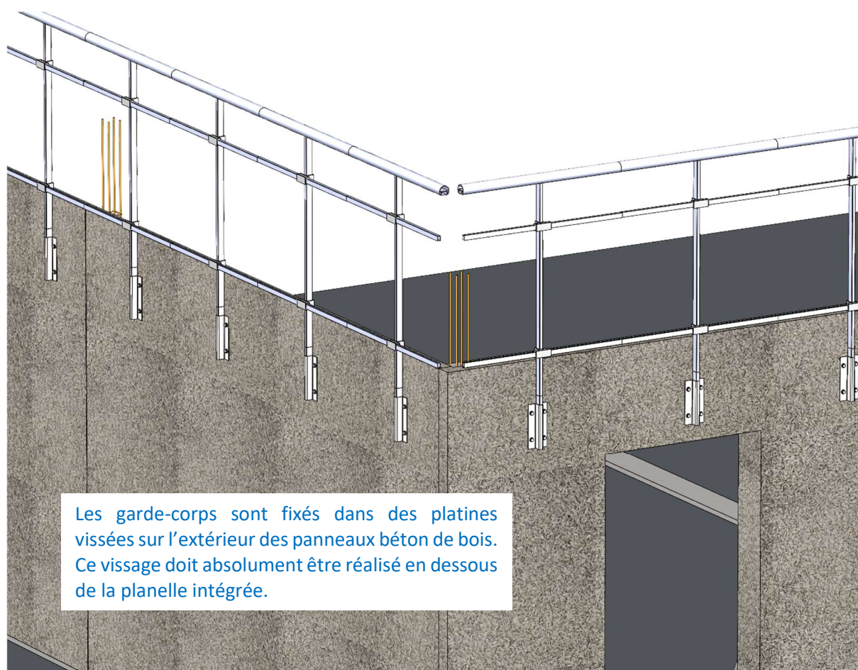
Figure A38 : Mise en place d'une protection collective par garde-corps
