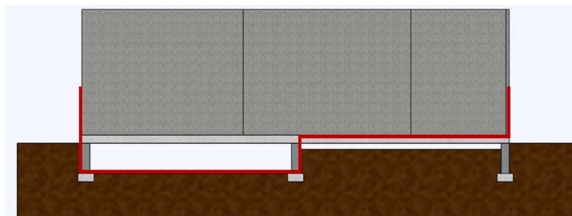
Figure A06 : Protection contre les termites – schéma de principe avec barrière continue
