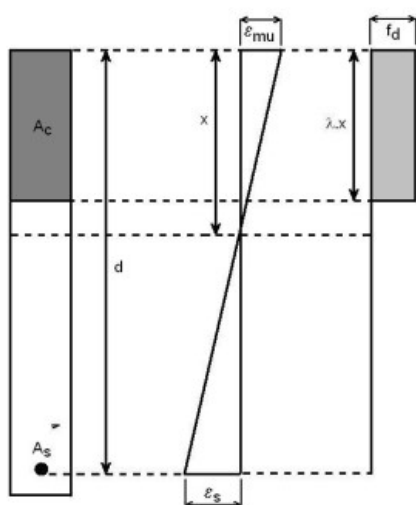
Figure A07-2 : Relation contrainte-déformation du remplissage – diagramme rectangle
