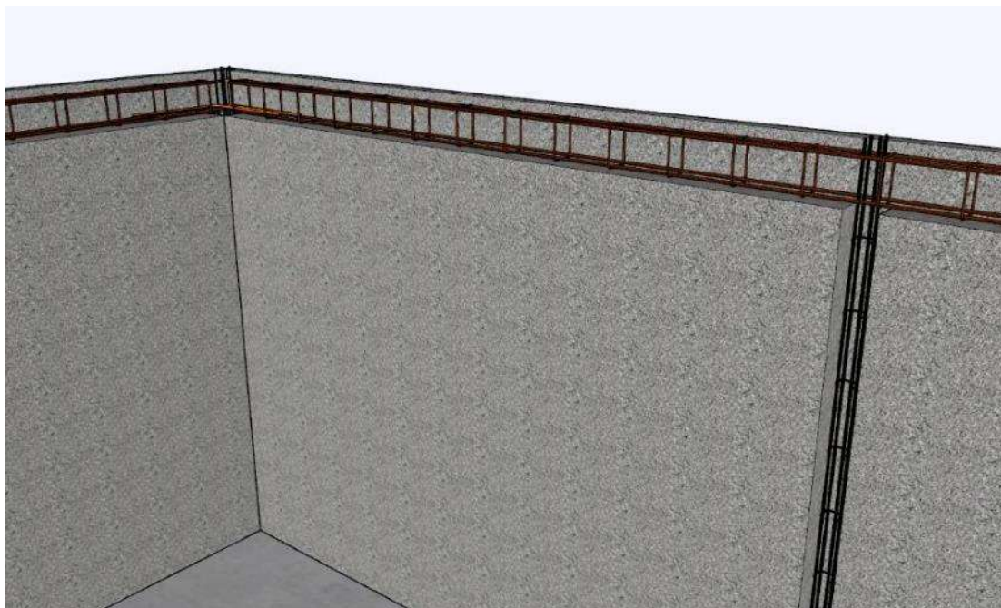
Figure A10 : Vue de principe des armatures de chaînages verticaux et horizontaux
