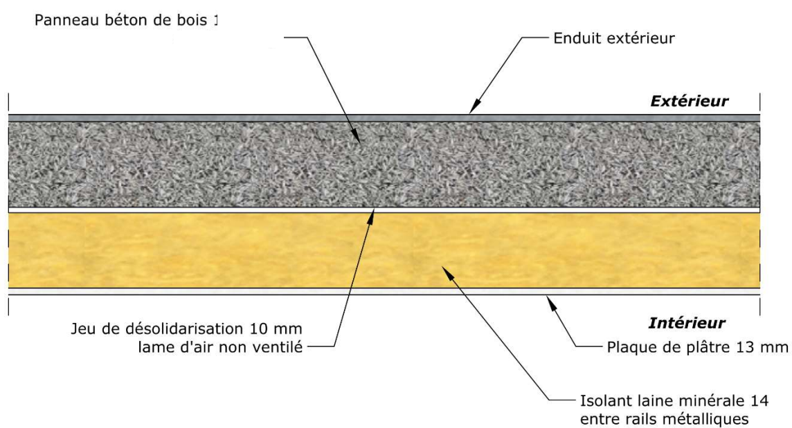
Figure A39 : Exemple partie courante Panneau avec enduit extérieur
