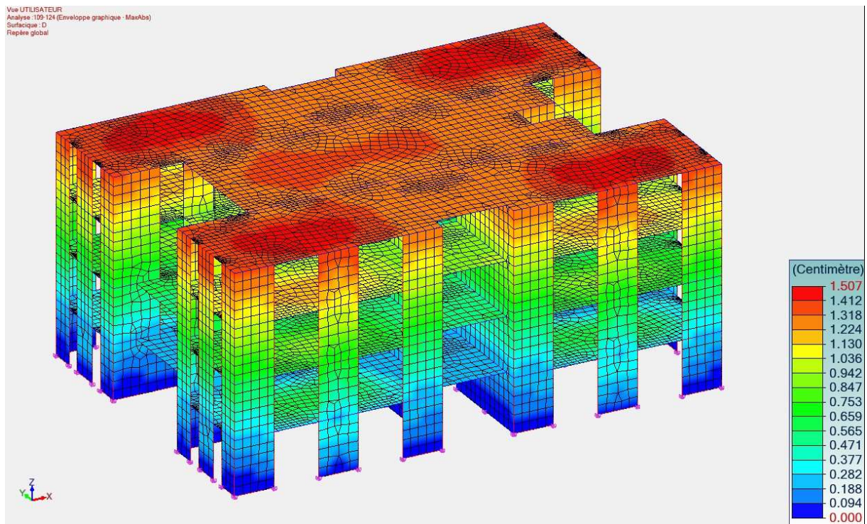
Fig. 17 – Modèle béton de bois CS2 – Déformée globale D
