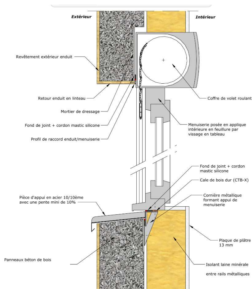
Figure A34 : Intégration des coffres et demi-coffres de volets roulants
