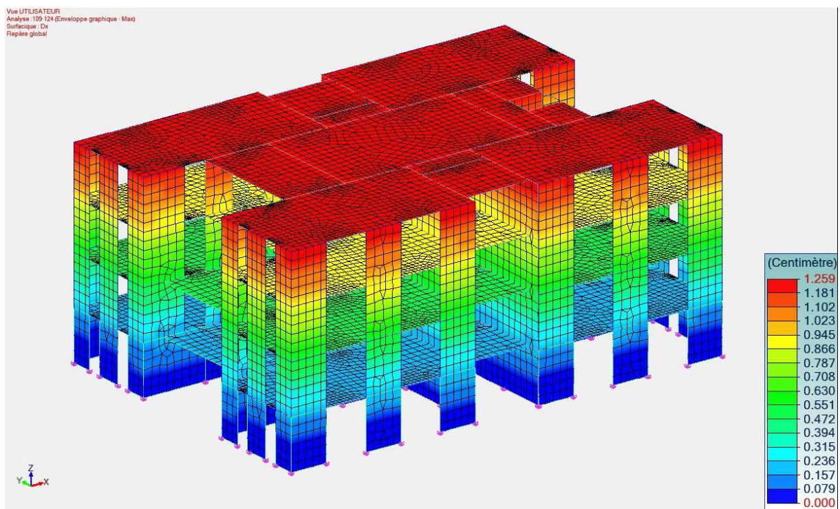
Fig. 18 – Modèle béton de bois CS2 – Déformée Dx selon direction X
