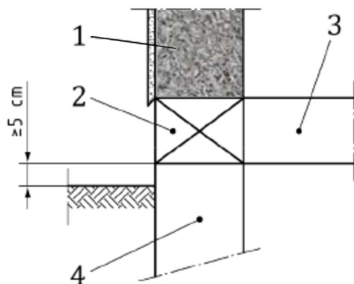
Figure A02 : Disposition anti-capillarité – solution 1 avec chaînage béton armé si soubassement en maçonnerie
