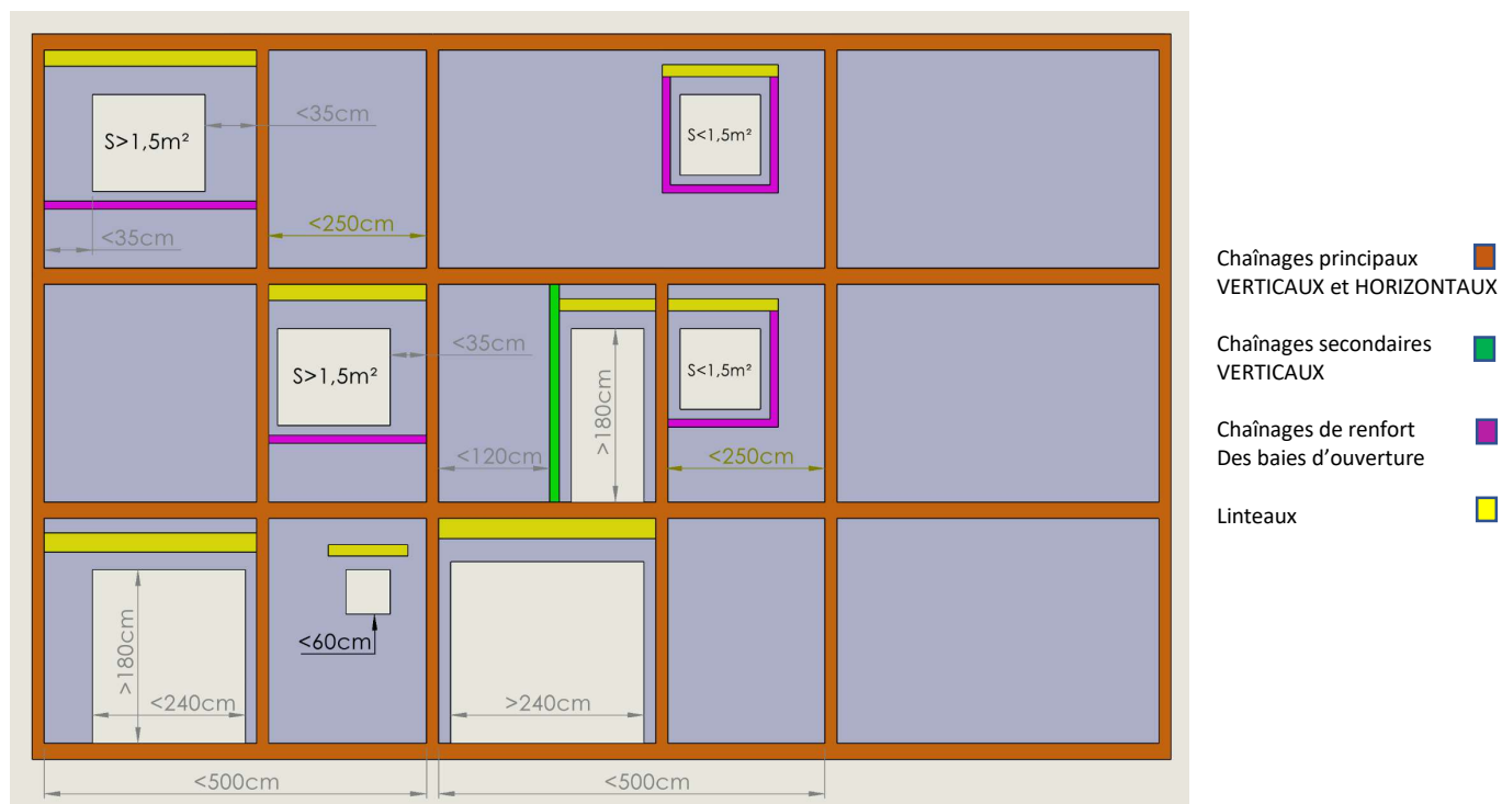
Figure A29 : Dispositions de principe des chaînages pour les configurations D, E et F – hors analyse de structure ou exigences particulières :
