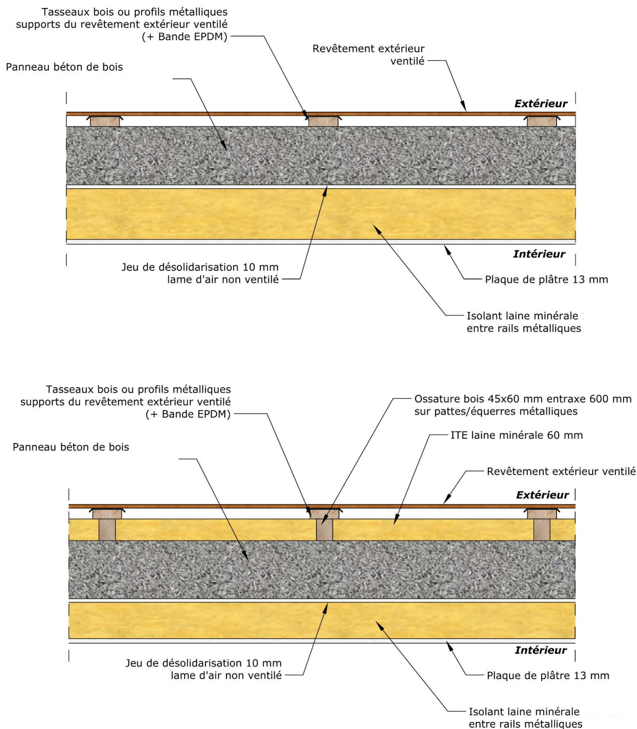
Figures A40 : Exemple partie courante Panneau avec bardages
