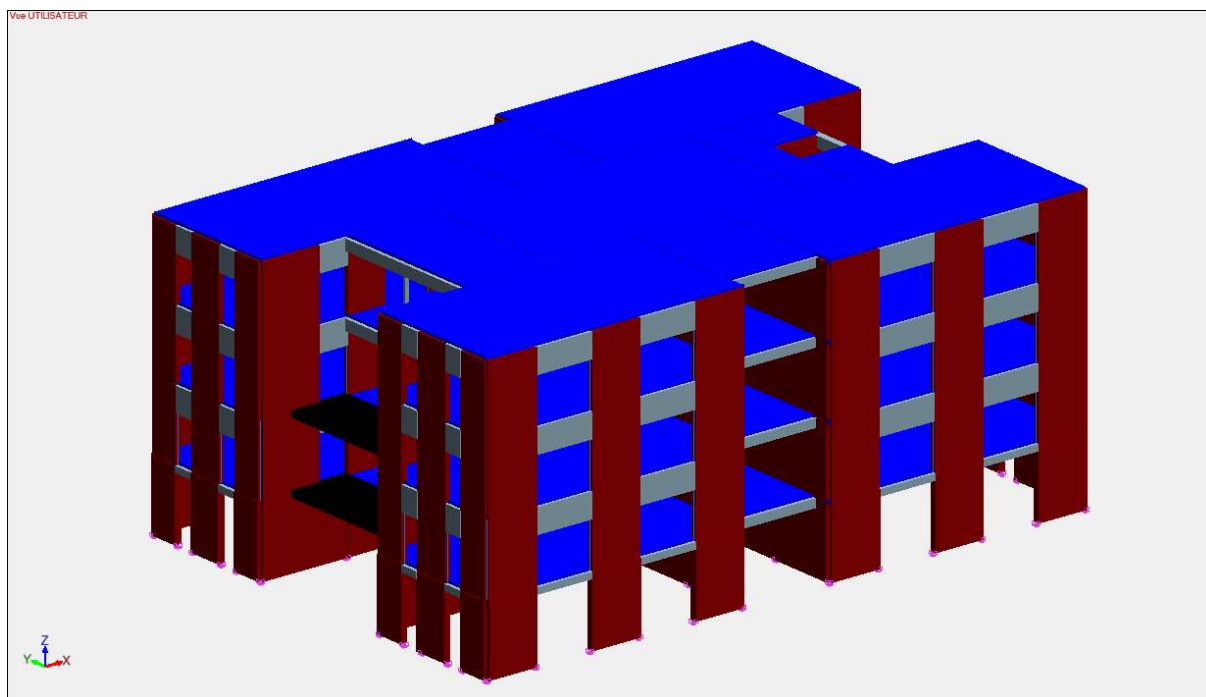
Fig. 5 – Modèle béton de bois CS2 - Axonométrie 1
