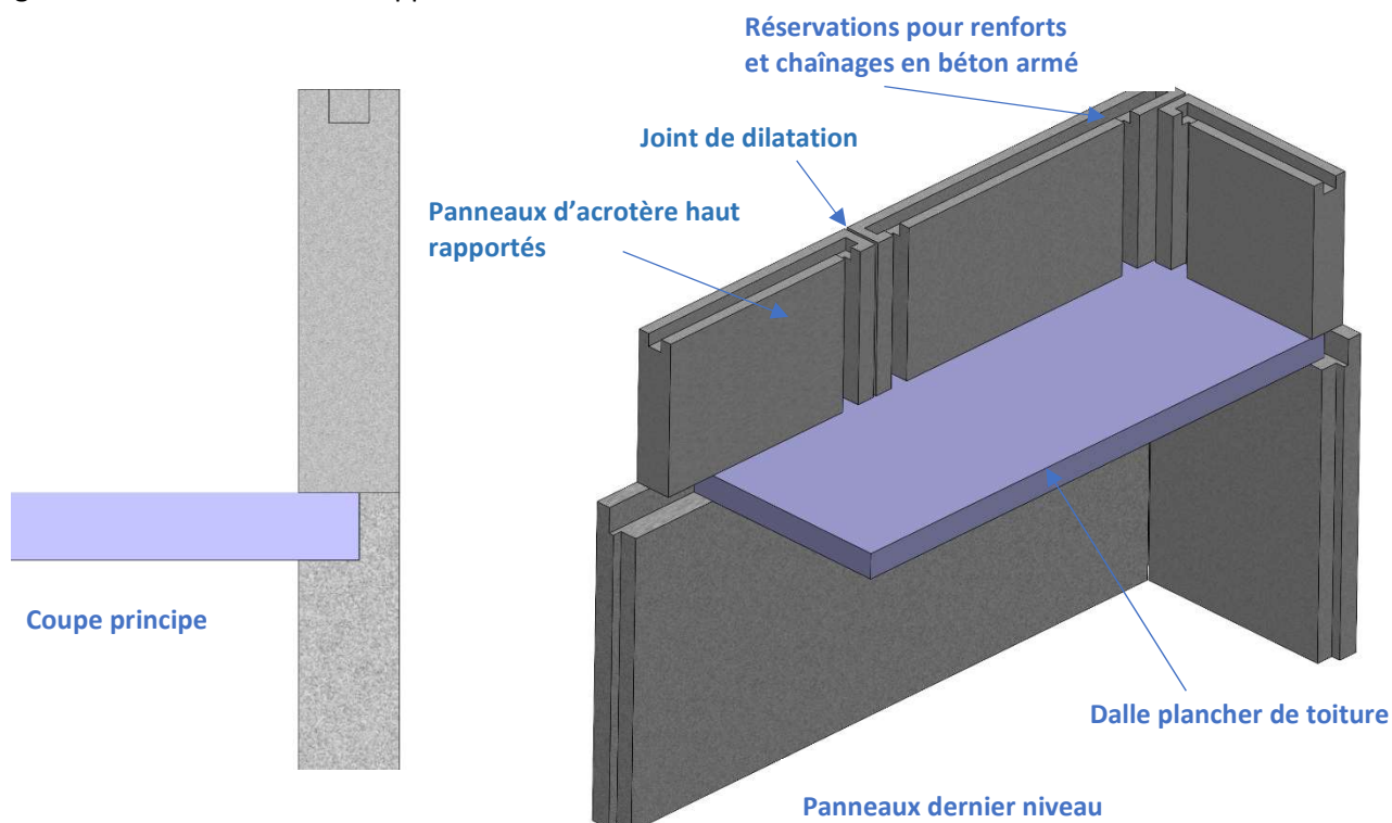
Figure A25-C : Acrotère haut rapporté sur dalle toiture
