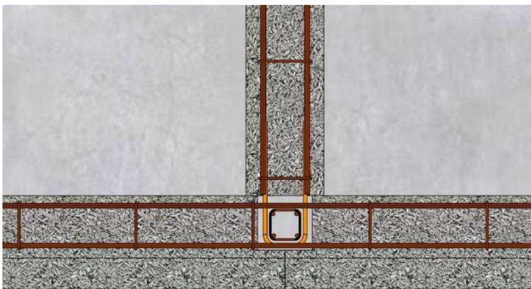
Figure A17 : Continuité des armatures de chaînages horizontaux avec équerres – Liaison refend
