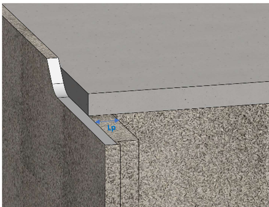
Figure A31 : Appui des planchers sur mur CS2 TimberRoc
