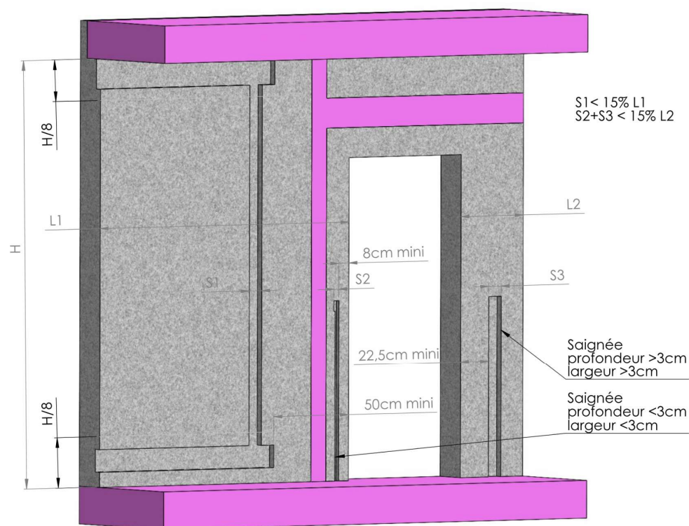
Figure A30 : Exemples de saignées dans un panneau béton de bois TimberRoc
