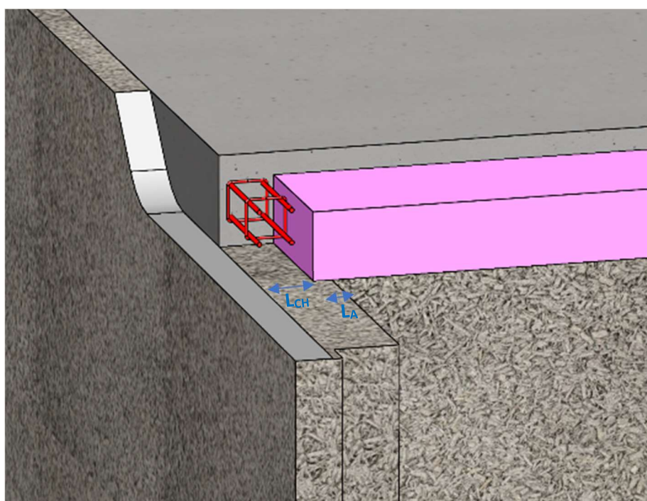
Figure A32 : Exemple d'appui de plancher préfabriqué
