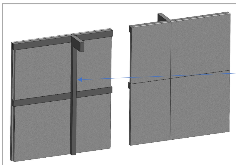
Figure A 36-A : Réalisation d'un poteau porteur en saillie sur 2 niveaux de panneaux CS2
