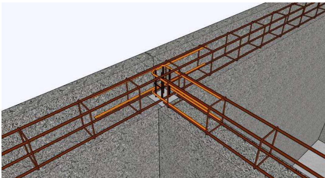
Figure A18 : Continuité des armatures de chaînages horizontaux avec équerres – Liaison refend / vue perspective
