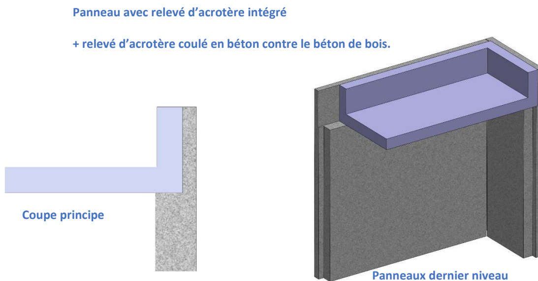
Figure A24-C : Acrotère bas mixte
