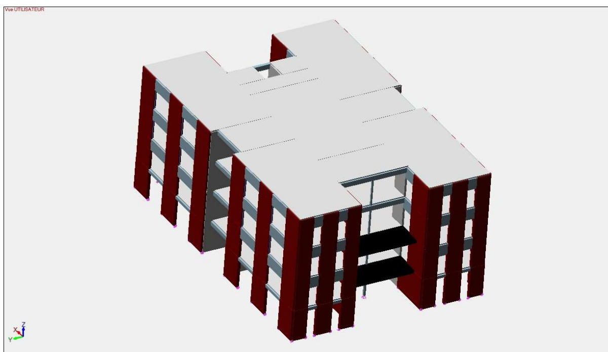
Fig. 13 – Modèle mixte (béton en gris et CS2 en rouge) - Axonométrie 2
