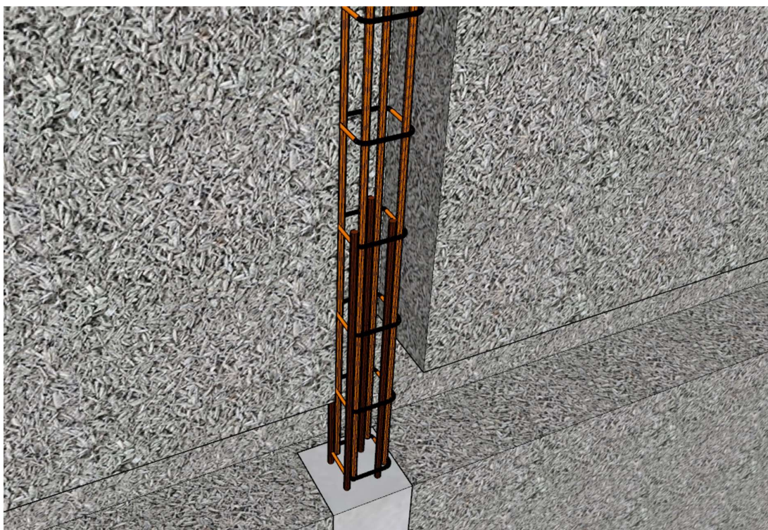
Figure A11 : Continuité des armatures de chaînages verticaux
