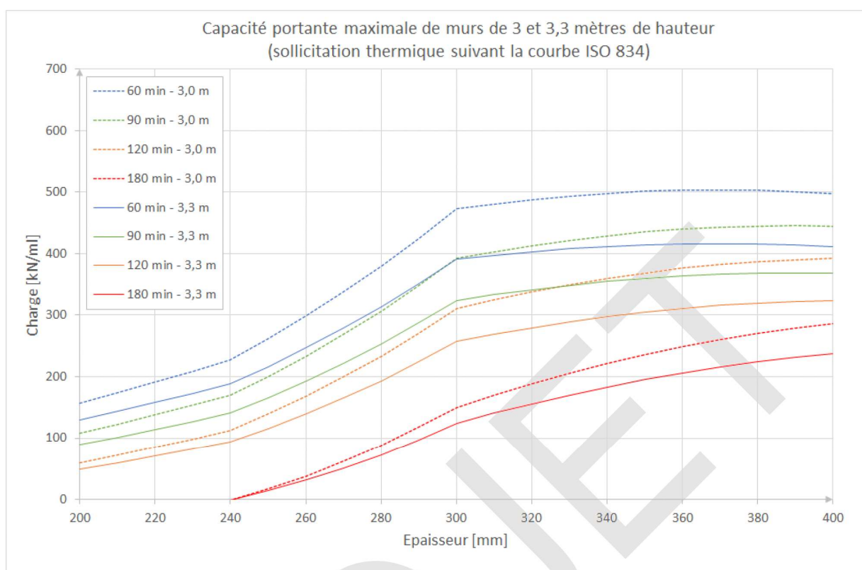
Figure 5.2 : Capacité portante des murs porteurs considérés selon l'épaisseur et la performance au feu recherchée
