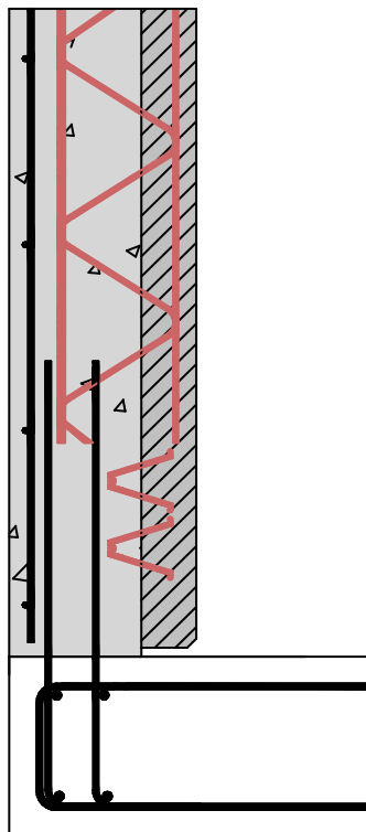
FIGURE 30 Liaison en pied (rotulée)
