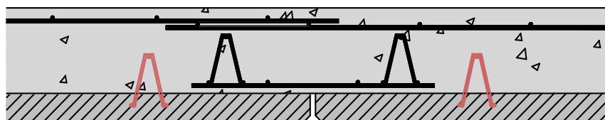
FIGURE 23 Liaison droite (rotulée)
