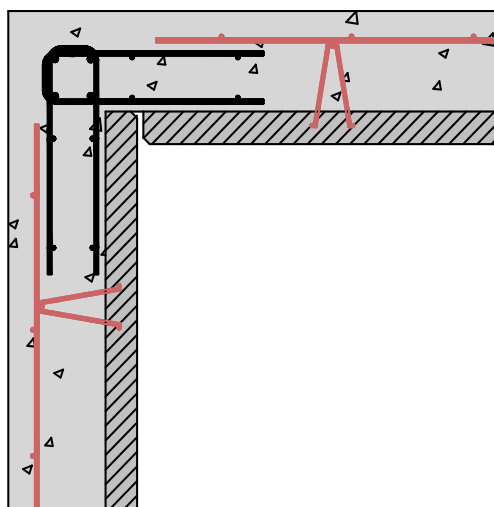
FIGURE 8 Liaison d'angle (couturée)
