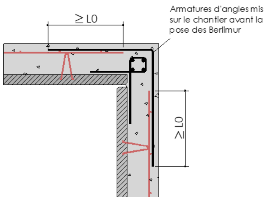
FIGURE 10 Liaison d'angle (encastrée coté intérieur)
