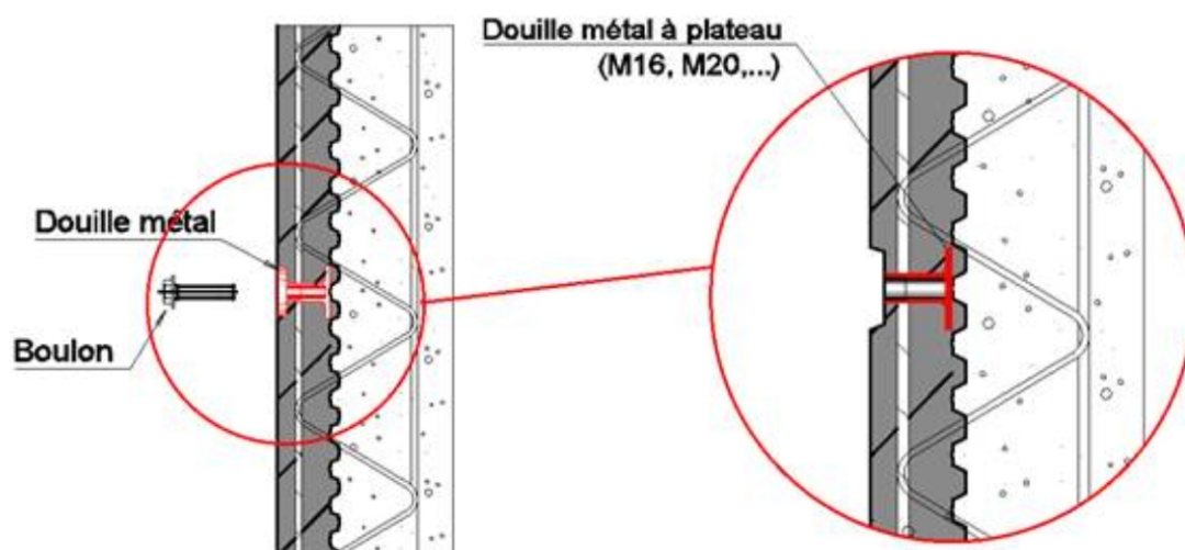
FIGURE 5 Douilles métal
