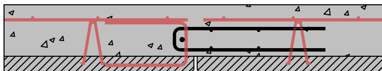
FIGURE 13 Liaison d'angle biaise (rotulée)
