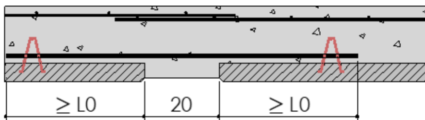
FIGURE 25 Liaison droite (encastée)
