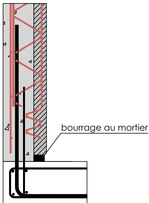
FIGURE 29 Liaison en pied (encastrée côté intérieur)
