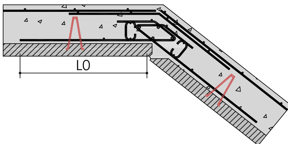
FIGURE 27 Liaison d'angle biaise (encastrée)
