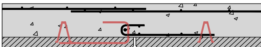
FIGURE 24 Liaison droite (couturée)
