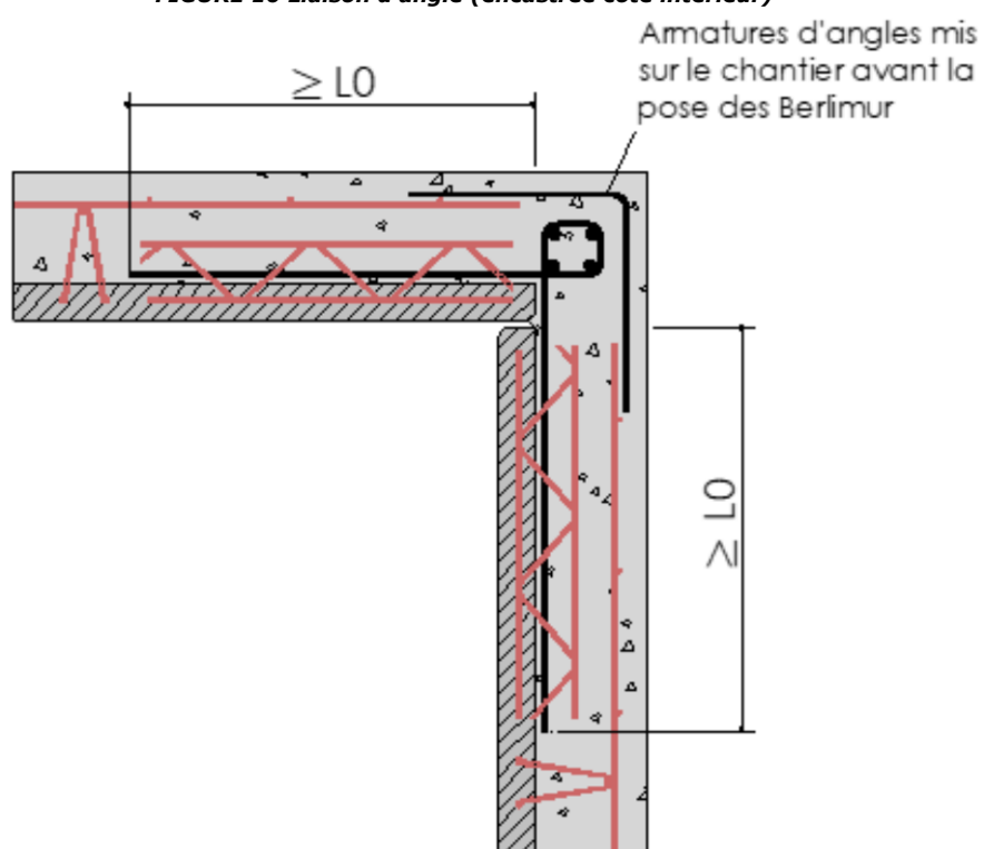
FIGURE 10 Liaison d'angle (encastrée coté intérieur)
