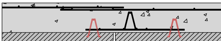
FIGURE 25 Liaison droite (encastée)
