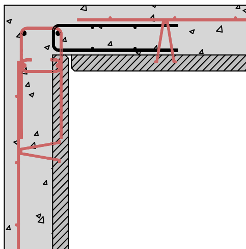
FIGURE 8 Liaison d'angle (couturée)
