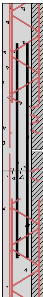
FIGURE 18 Liaison horizontale (encastrée)
