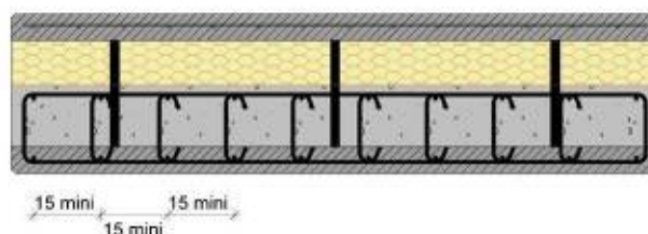
Figure g - Armatures d'éclissage
